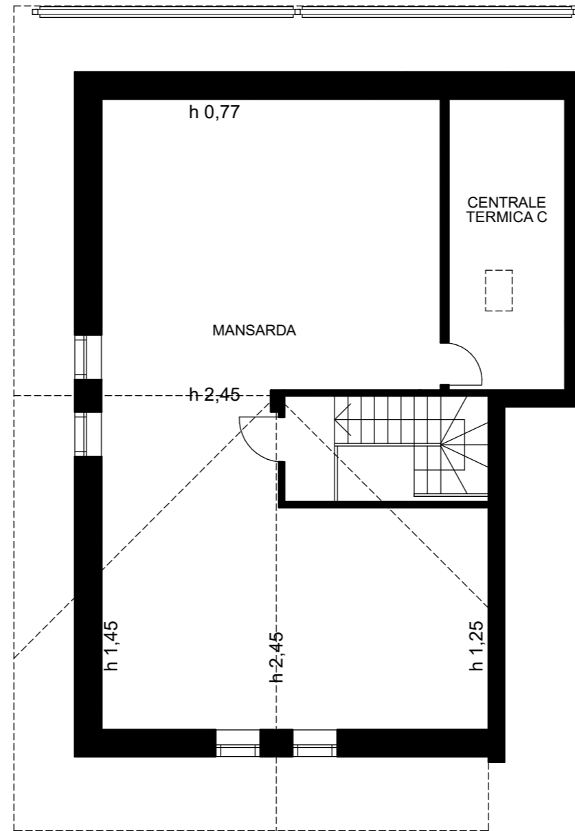
PIANO SOTTOTETTO
